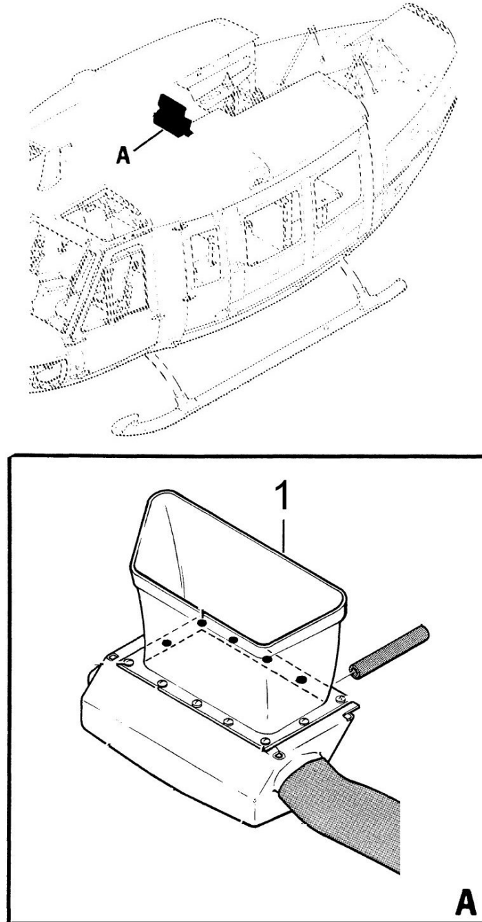
Figure 21-2 D212-725-1-949 Duct
